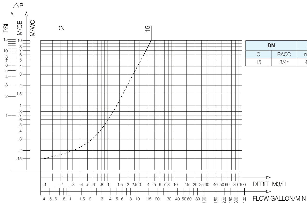
EA 251SPU - Abaque des pertes de charge
