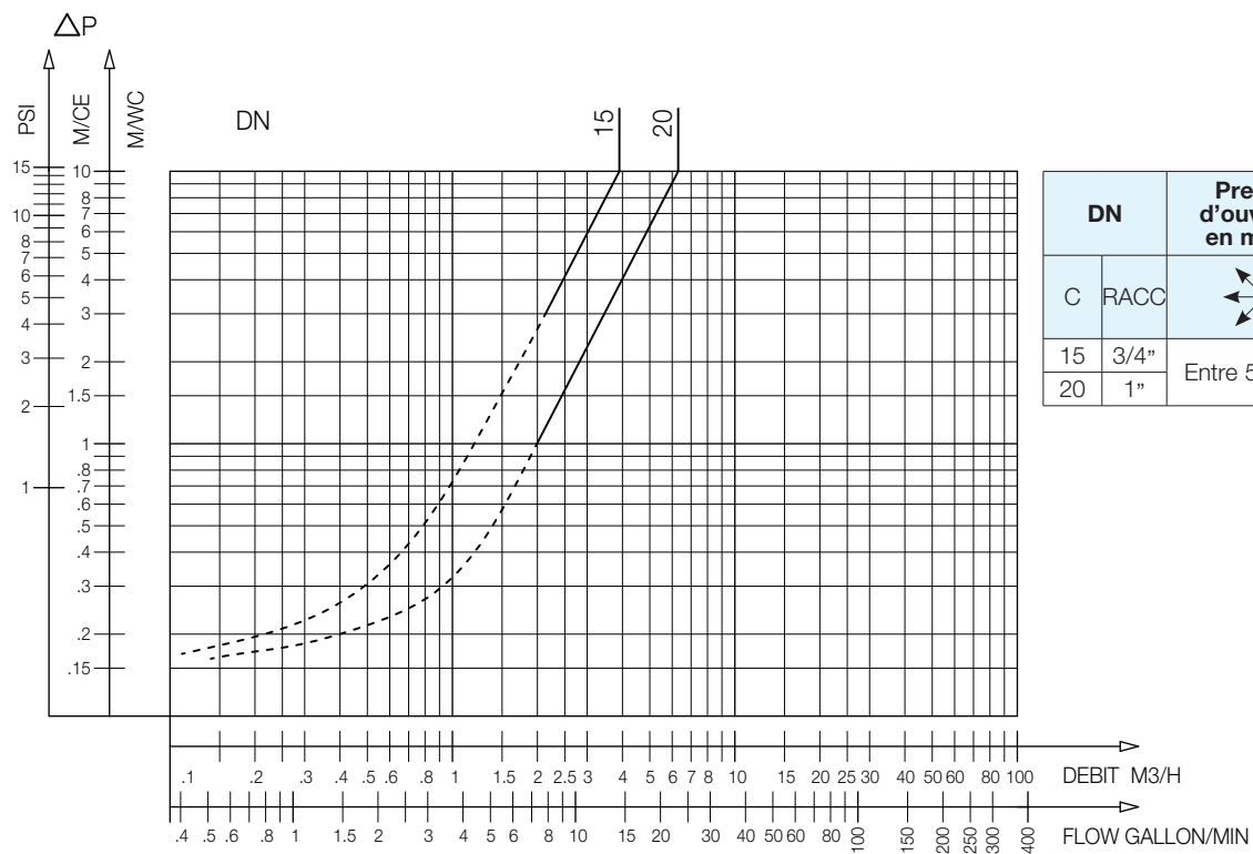
EA 251CC - Abaque des pertes de charge
